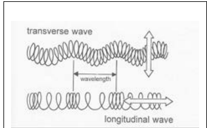
Fig. 2: transversal/longitudinal wave. Dubeck 9
